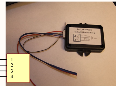
иммитатор шины CAN BMW E series
